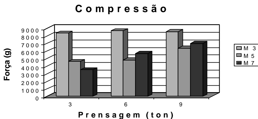
Figura 1 - Avaliação comparativa da força de compressão dos blocos de café nos níveis P3, P6 e P9 para as moagens fina, média e grossa.
