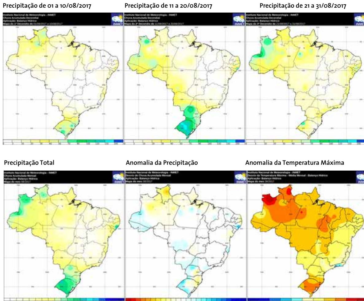
Figura 19 - Precipitação decenal, precipitação total, anomalia da precipitação e da temperatura máxima média em agosto de 2017
