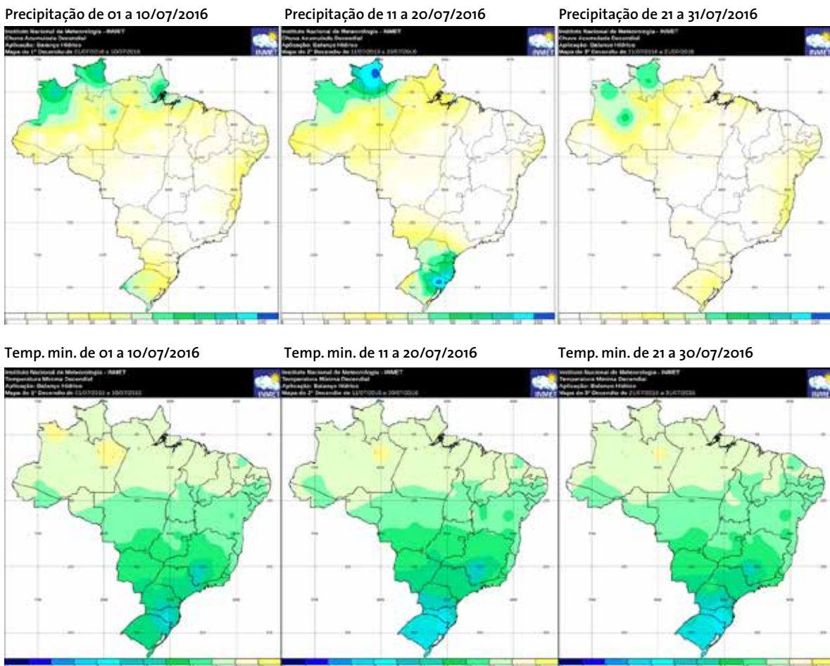
Figura 6 – Precipitação e temperatura mínima média decenal, precipitação total, anomalia da precipitação e temperatura mínima média, em julho de 2016
