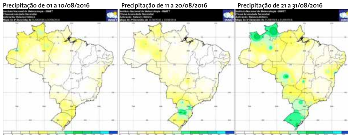
Figura 7 - Precipitação decendial, precipitação total, anomalia da precipitação e da temperatura máxima média em agosto de 2016
