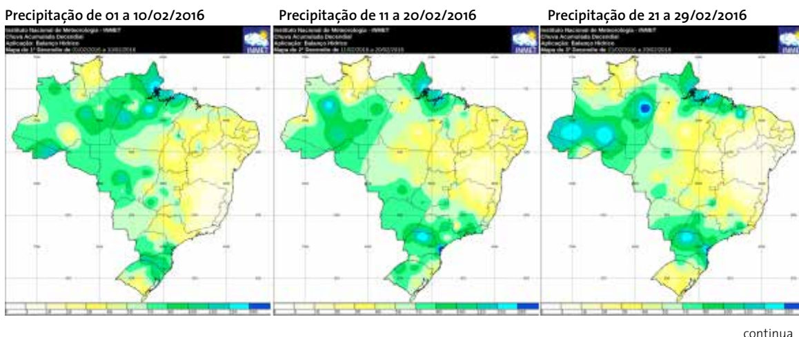
Figura 1 - Precipitação decendial, precipitação total, anomalia da precipitação e da temperatura máxima média em fevereiro de 2016
