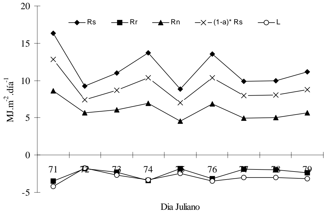
Figura 17 – Componentes do balanço de radiação ( \text{MJ}/\text{m}^2.\text{dia} ) em uma cultura de café, Coffea arabica , Catuaí-Vermelho. São Miguel do Anta, MG, 12/03/2004 – 20/03/2004.
