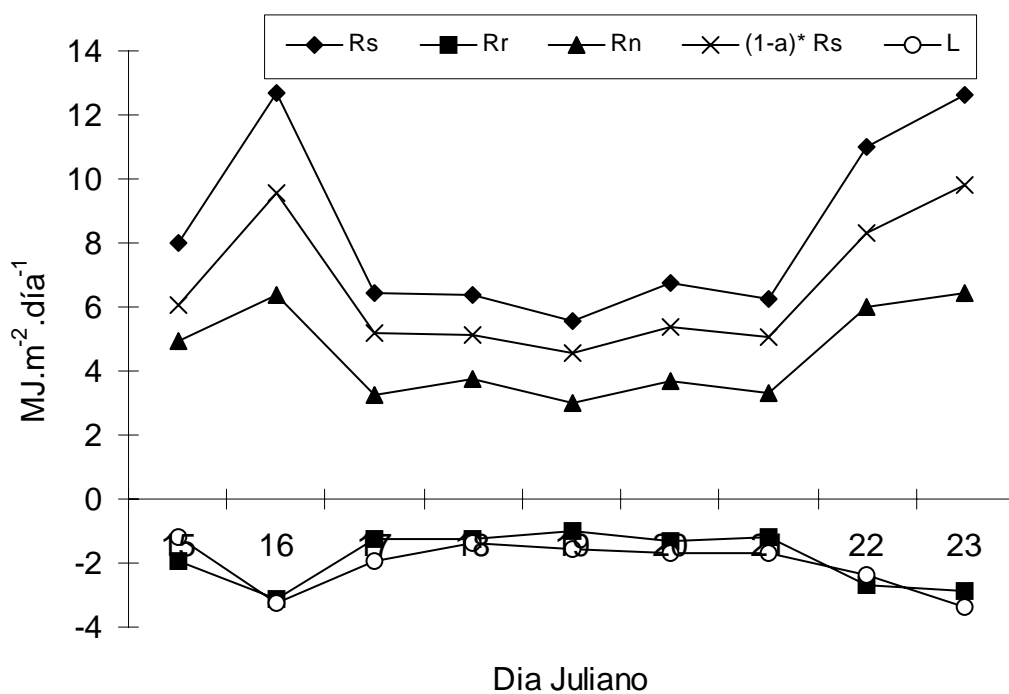
Figura 16 – Componentes do balanço de radiação ( \text{MJ}/\text{m}^2.\text{dia} ) em uma cultura de café, Coffea arabica , Catuaí-Vermelho. São Miguel do Anta, MG, 15/01/2004 – 23/01/2004.
