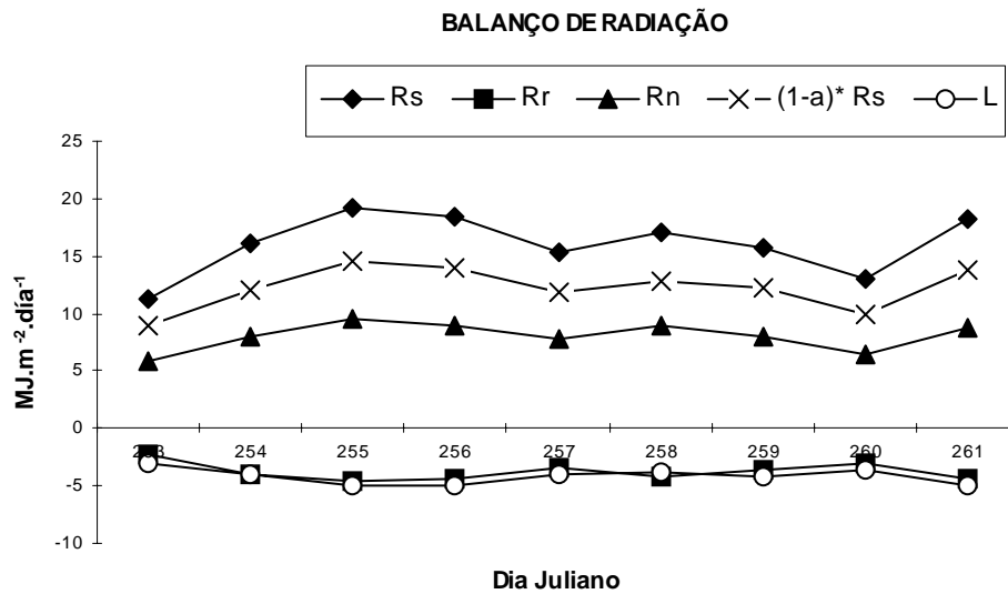
Figura 18 – Componentes do balanço de radiação (MJ/m 2 .dia) em uma cultura de café, Coffea arabica , Catuaí-Vermelho. São Miguel do Anta, MG, 10/09/2004 – 18/09/2004.
