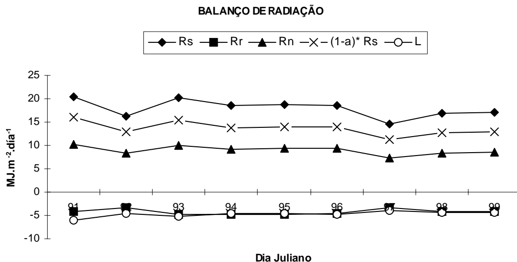
Figura 20 – Componentes do balanço de radiação ( \text{MJ}/\text{m}^2.\text{dia} ) em uma cultura de café, Coffea arabica , Catuaí-Vermelho. São Miguel do Anta, MG, 01/04/2005 – 09/04/2005.
