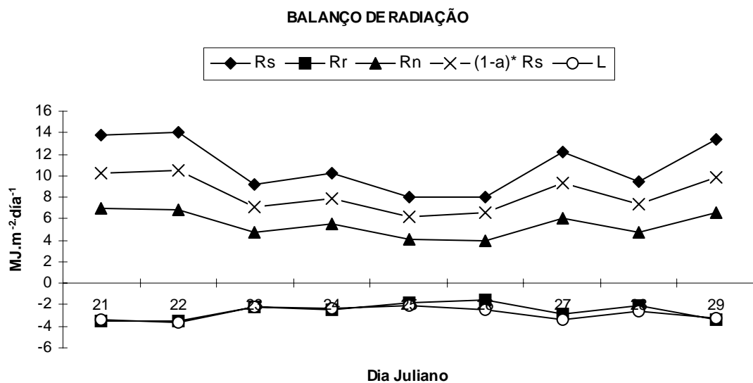
Figura 19 – Componentes do balanço de radiação (MJ/m 2 .dia) em uma cultura de café, Coffea arabica , Catuaí-Vermelho. São Miguel do Anta, MG, 21/01/2005 – 29/01/2005.
