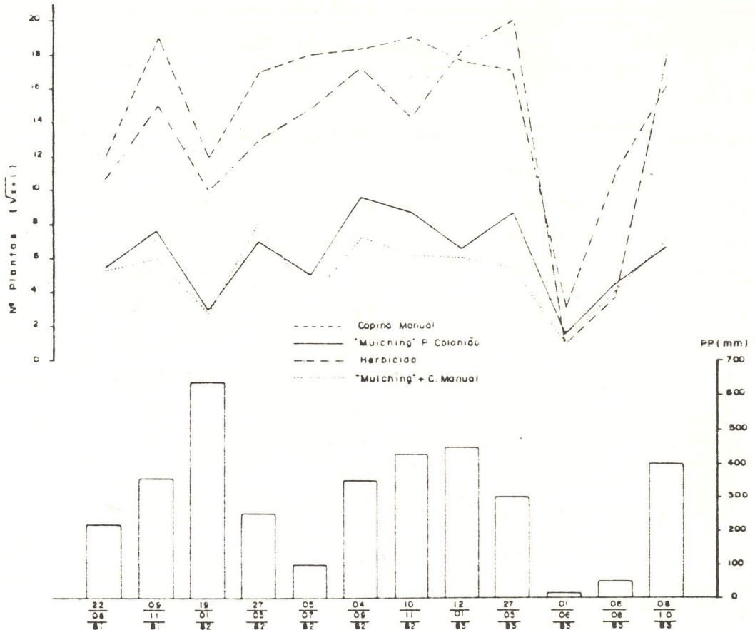
FIGURA 1. Incidência das Plantas Daninhas ( \sqrt{x+1} ) em Função dos Métodos de Controle e de Precipitação (mm de Chuva), nas Doze Épocas de Aplicação dos Tratamentos. Rio Branco, Ac. 1984.
