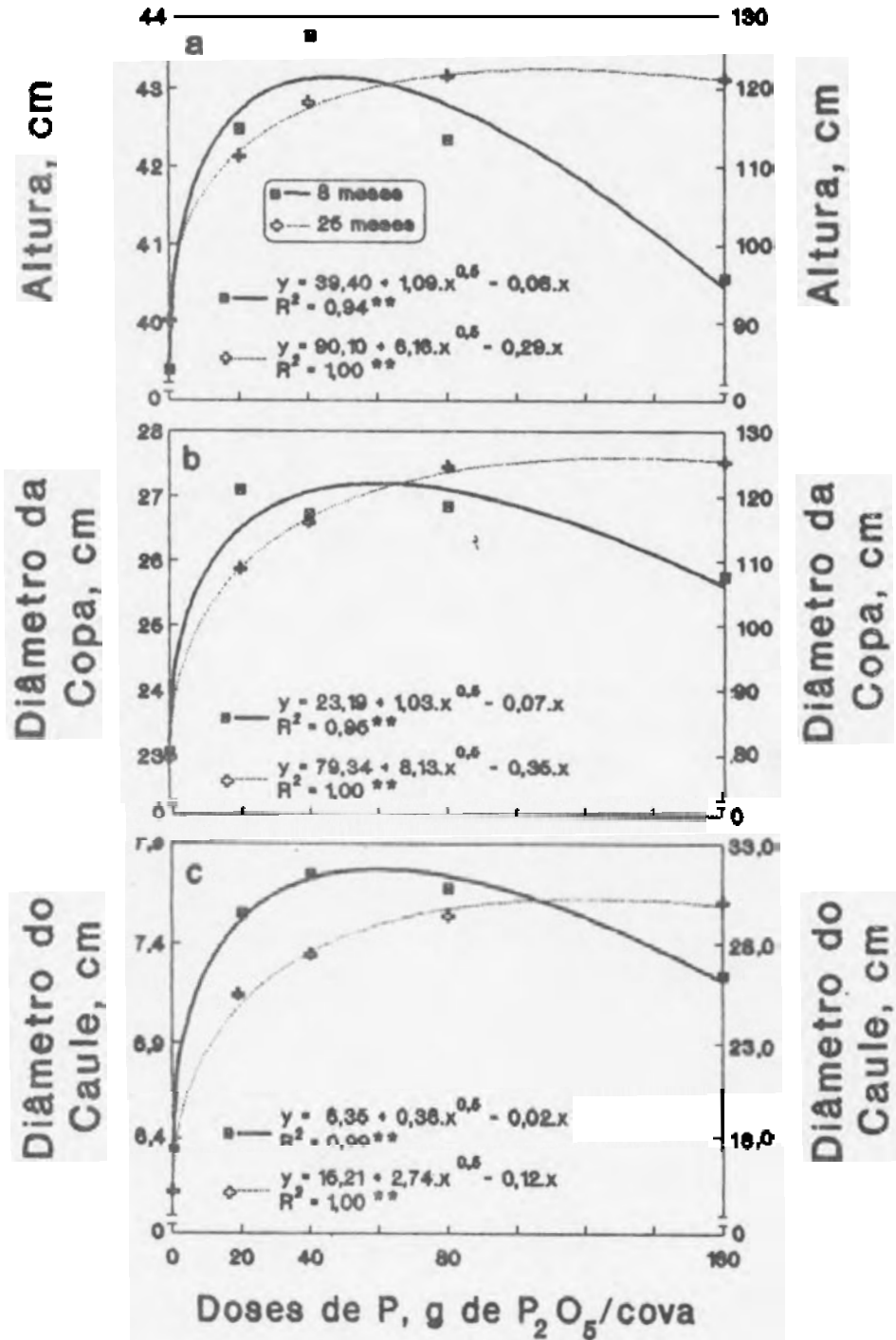
Figura 5. Altura (a), diâmetro da copa (b) e diâmetro do caule (c) de cafeeiros pré-colonizados com FmVA em função do P aplicado na cova, aos 8 (escala à esquerda) e 25 meses (escala à direita) pós-transplante para o campo. ^{**} Regressão significativa à 1% pelo teste de F de Snedecor.
