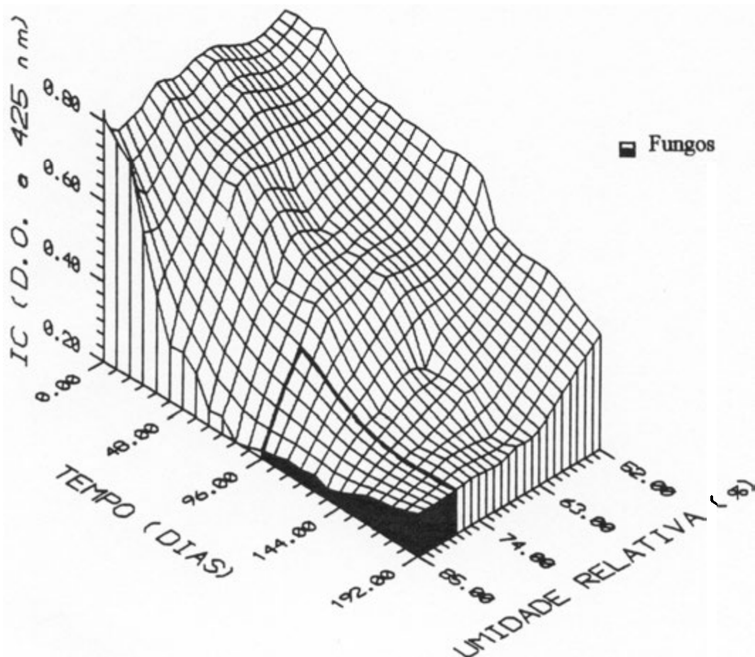
FIGURA 18 - Comportamento dos Índices de Coloração (IC) de Grãos de Café Beneficiados e Armazenados em Temperatura de 20°C e Diferentes Umidades Relativas, Durante o Período de Armazenamento, UFLA, Lavras - MG, 1995.
