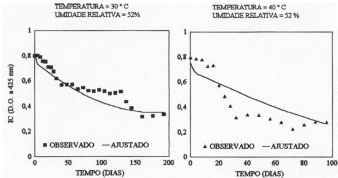
FIGURA 25 - Valores dos Índices de Coloração Obtidos Experimentalmente e Calculados Através do Modelo Ajustado para 52% de Umidade Relativa e Temperaturas de 30 e 40° C. UFLA, Lavras - MG, 1995.
