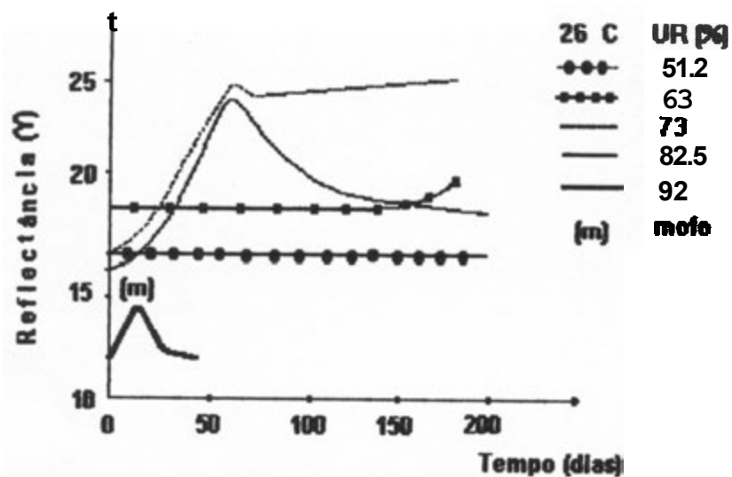
FIGURA 1 - Evolução da Reflectância de Grãos de Café, em Função do Tempo de Armazenagem, em Diferentes Umidades Relativas, (Santos et al., 1971).
