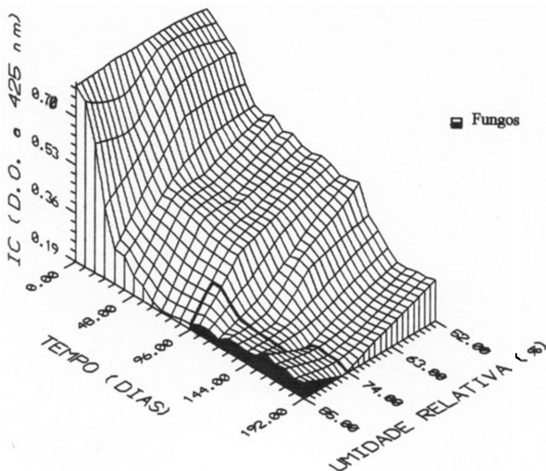
FIGURA 19 - Comportamento dos Índices de Coloração (IC) de Grãos de Café Beneficiados e Armazenados em Temperatura de 30°C e Diferentes Umidades Relativas, no Decorrer do Período de Armazenamento, UFLA, Lavras -MG, 1995.
