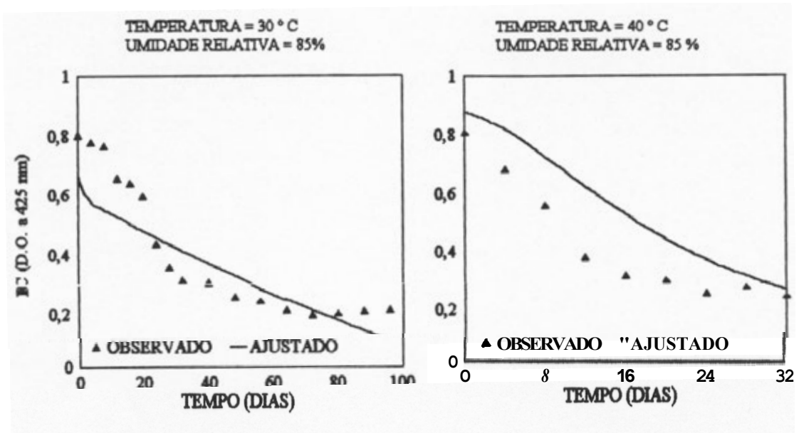
FIGURA 31 - Valores dos Índices de Coloração obtidos experimentalmente e calculados através do modelo ajustado para 85% de umidade relativa e temperaturas de 30 e 40° C, UFLA, Lavras - MG, 1995.
