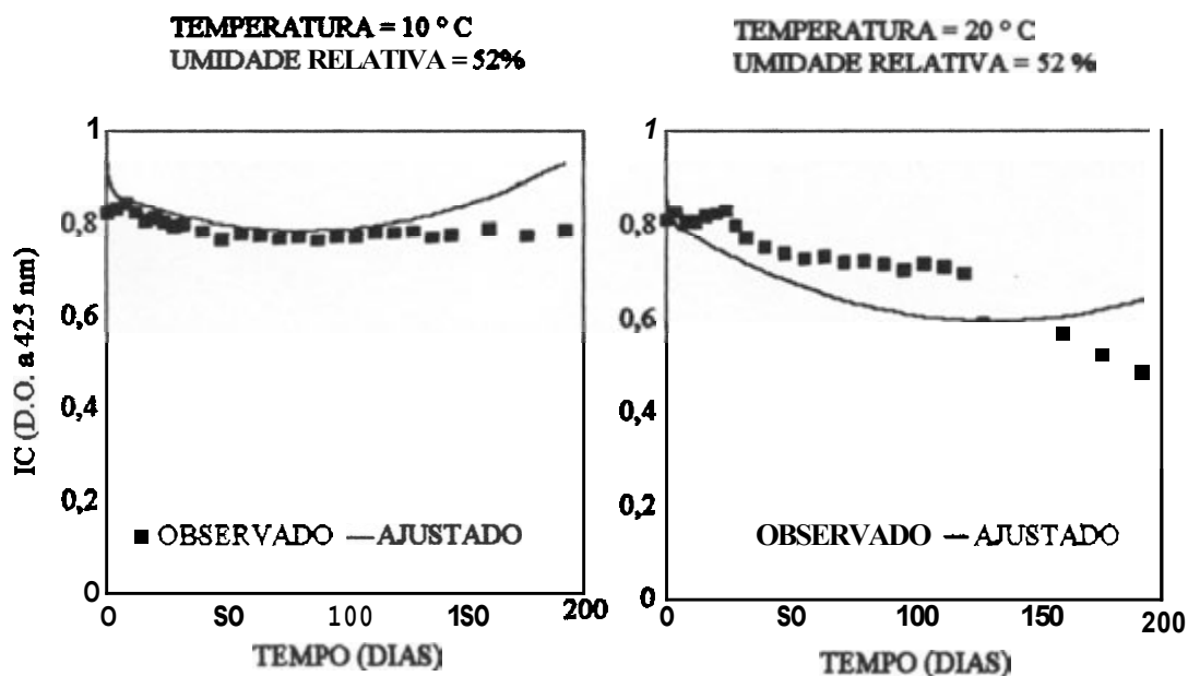
FIGURA 24 - Valores do Índice de Coloração Obtidos Experimentalmente e Calculados Através do Modelo Ajustado para 52% de Umidade Relativa e Temperaturas de 10 e 20° C, UFLA, Lavras - MG, 1995.
