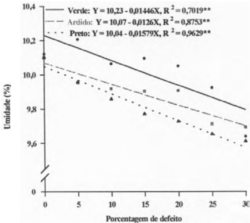
FIGURA 9. Representação gráfica e equações de regressão dos teores de umidade em função das quantidades de inclusão dos defeitos “verde”, “ardido” e “preto”.
