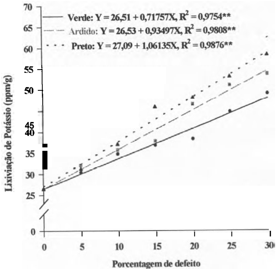
FIGURA 5. Representação gráfica e equações de regressão da lixiviação de potássio em função das quantidades de inclusão dos defeitos “verde”, “ardido” e “preto”
