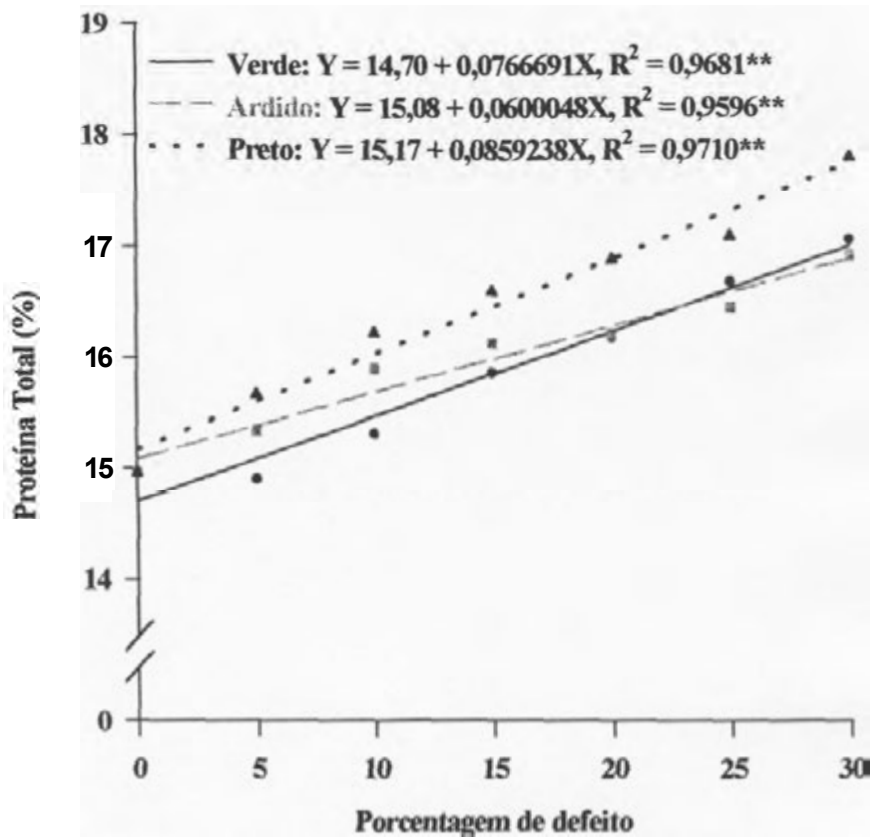
FIGURA 21. Representação gráfica e equações de regressão dos teores de proteínea total em função das quantidades de inclusão dos defeitos “verde”, “ardido” e “preto”
