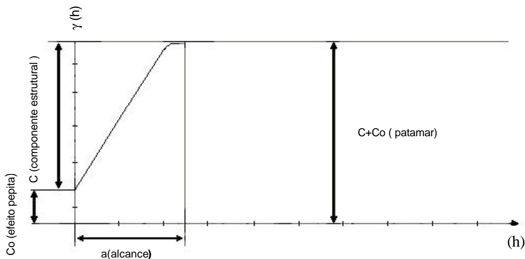
Figura 7- Semivariograma e seus componentes
